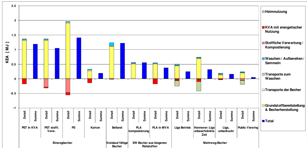
Abbildung 46: Sensitivitätsbetrachtungen Ligabetrieb und Public Viewing für KEA: BELLAND®Material zu 50% Rezyklat, PLA mit Kompensation der CO 2 -Emissionen, PS mit stofflicher Verwertung, alle MW Szenarien waschen mit Ökostrom, Ligabetrieb einbedruckte Becher ohne Berücksichtigung der Heimnutzung.
