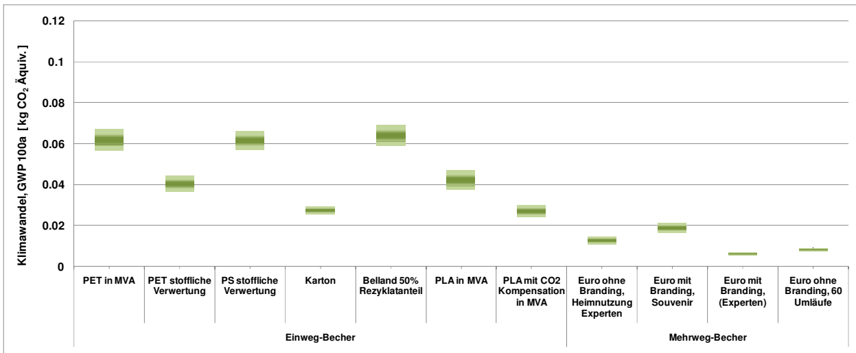
Abbildung 6: Sensitivitätsbetrachtung der Auswirkungen auf das Klima von verschiedenen Getränkebechern mit Angabe der Fehlerbandbreiten
