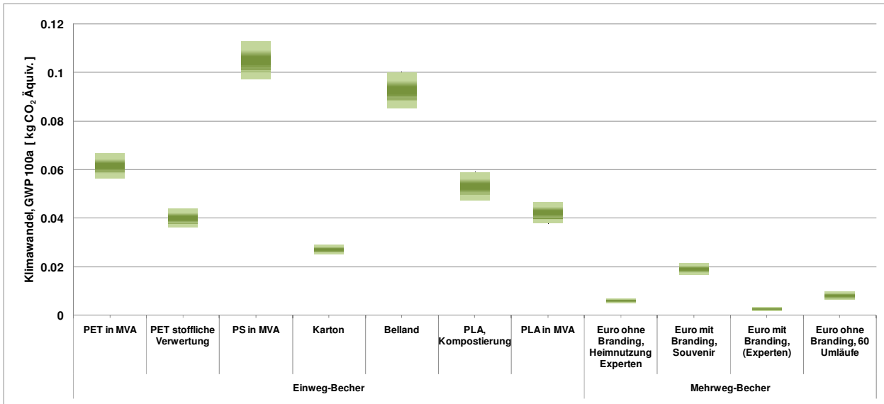
Abbildung 3: Auswirkungen auf das Klima der verschiedenen Getränkebecher mit Angabe der Fehlerbandbreiten
