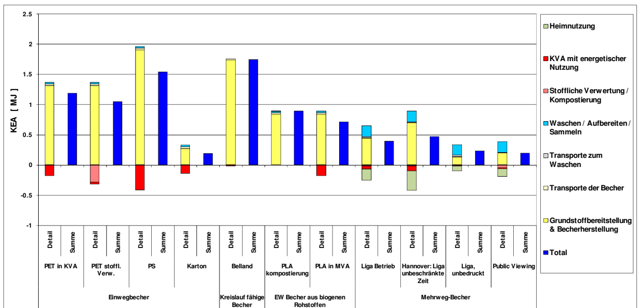
Abbildung 40: Detailanalyse der Ergebnisse Ligabetrieb und Public Viewing mit Angaben zu den verschiedenen Prozessen für KEA
