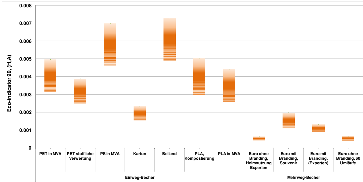
Abbildung 2: Umweltauswirkungen der verschiedenen Getränkebecher bewertet mit der Methode Eco-indicator 99 HA mit Angabe der Fehlerbandbreiten
